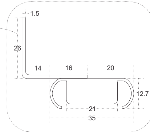
Échelle de l'équerre / Bracket scale 1:1 (100 %)
